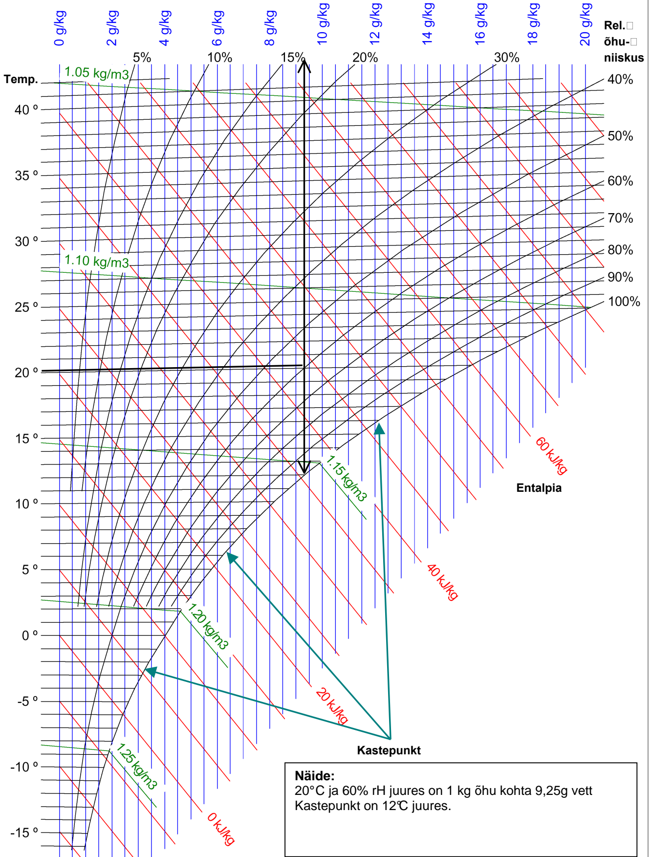
Mollieri Hx-diagramm õhurõhul 0,950 bar
